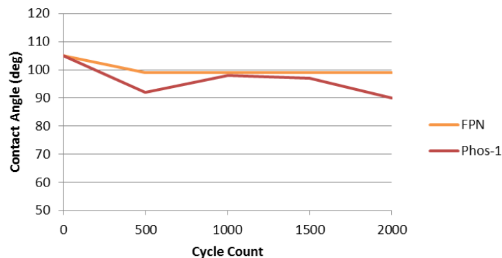
Abrasion - IPA
