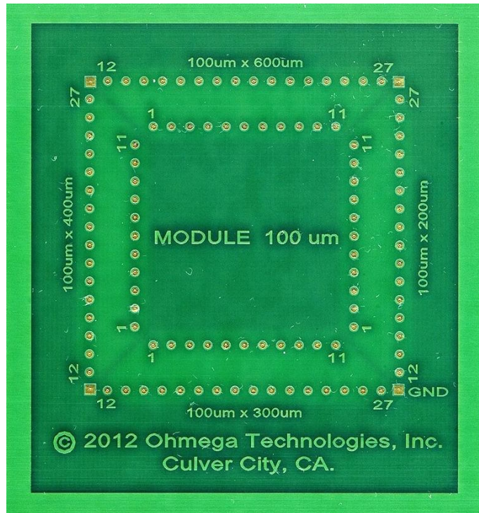
Top side
