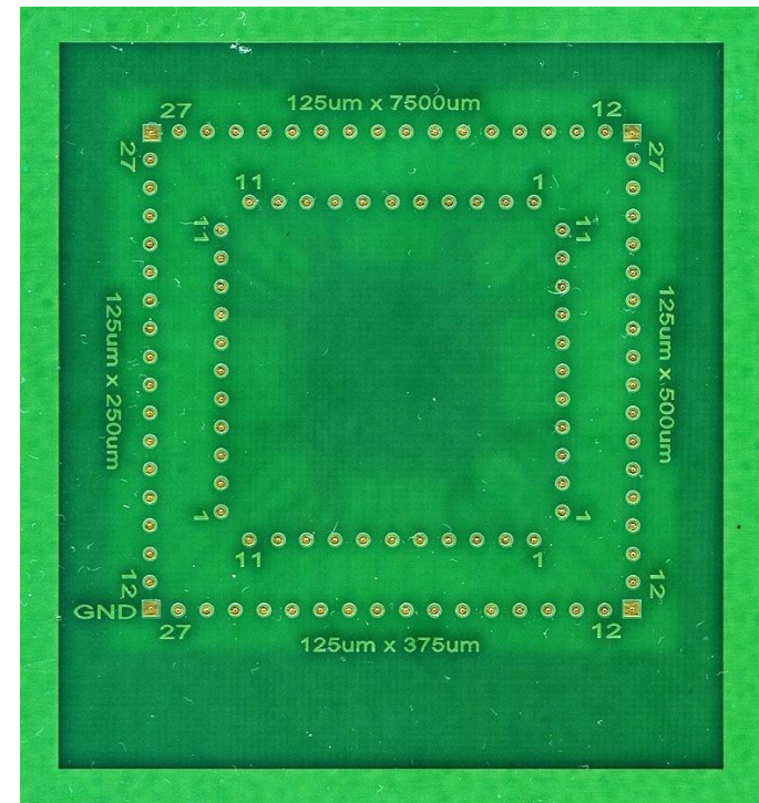
Bottom side
