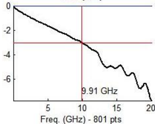
s21 (dB)
