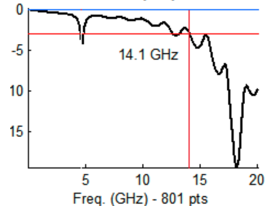
s21 (dB)
